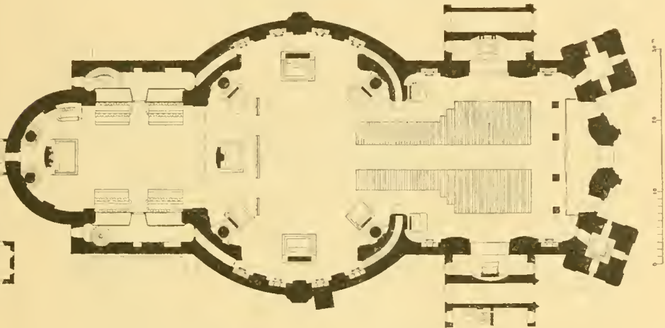
Fig. 95. Klosterkirche zu Wiblingen. Grundriss.
